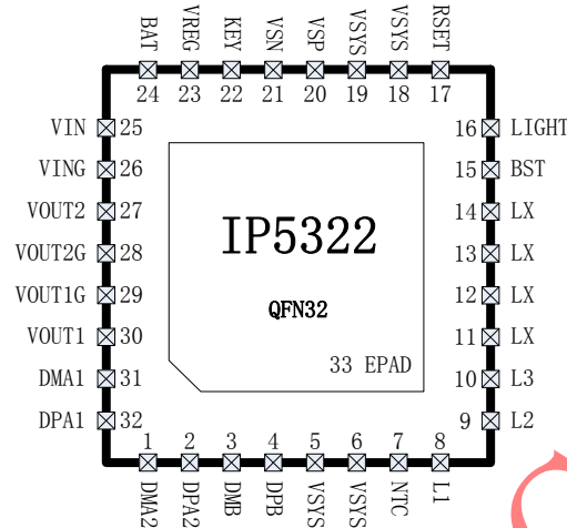
图 2 IP5322 引脚图
